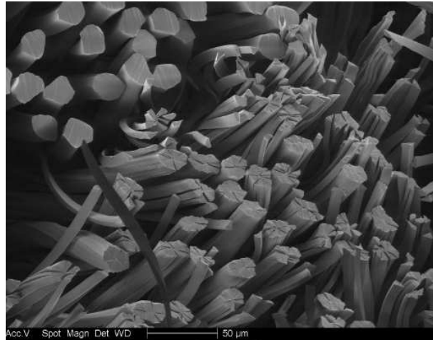
Figuur 1: Overzichtfoto van een topkwaliteit geweven microvezelmateriaal. Linksboven zijn de massieve kettingsdraden te zien, rechtsonder de microvezel inslagdraden. De meeste moedervezels (doorsnee 18 micrometer, dus officieel geen microvezel) zijn gesplitst in filamenten met een hoogte van 8 micrometer en een dikte van 5 micrometer (zie detail, onder). Dat zijn de daadwerkelijke microvezels. Deze foto's zijn gemaakt met een elektronenmicroscop door TNO, Rijswijk.
